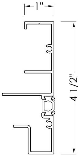
CW209 DOOR ADAPTER
